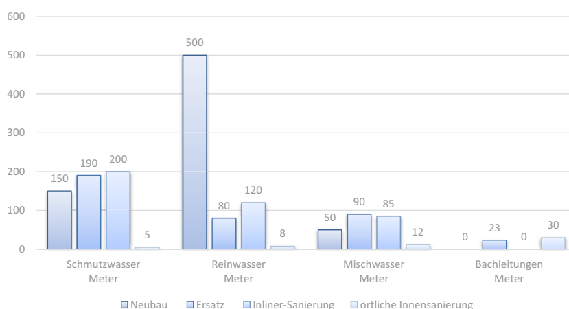
Abwassernetz erneuert und saniert 2024
