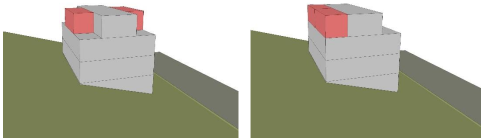
Abbildung 37: «Reguläre» Anordnung der Dachaufbauten beim Attikageschoss (links) sowie komplette hangseitige Anordnung der Dachaufbauten (rechts) (Quelle: EBP)
