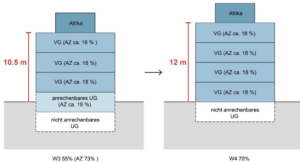
Abbildung 29 Aufhebung des anrechenbaren Untergeschosses am Beispiel der W3 55 % (neu: W4 70 %), die Aufhebung des anrechenbaren Untergeschosses wird auch in anderen Zonen vorgenommen (siehe Anhang A1) (Quelle: EBP)
